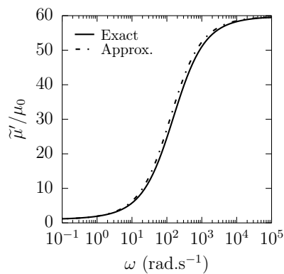
FIGURE 1 – Module viscoélastique d'un mélange de polymères
